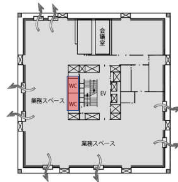
センターコア方式
