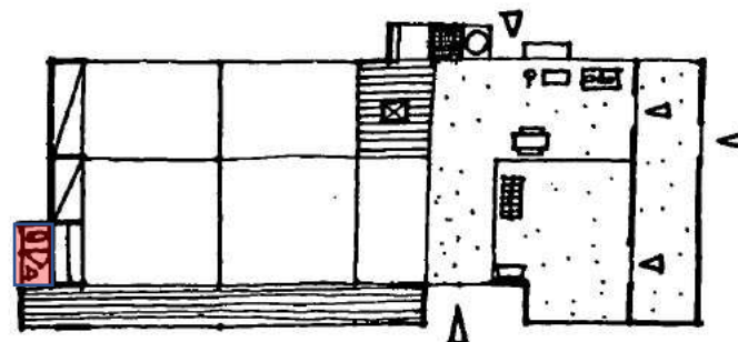
徳川時代 待 接待の家 ゲンカン・ナカノマ・オク・トコ・ベンゾが一体となって 接客空間をなす 千葉孝宣 勢お (昭和28年2月調査)
